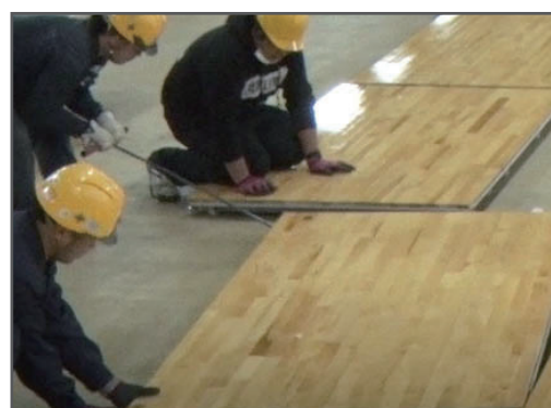
引き抜き工具にてパネルを引き抜く
