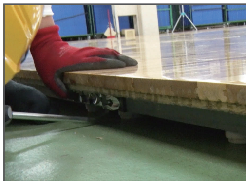
専用工具にてジョイント金具を解除
